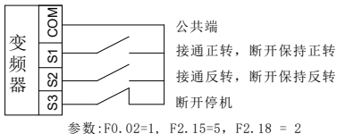
三线式控制模式 1
